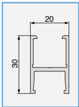
Jamb profile.
